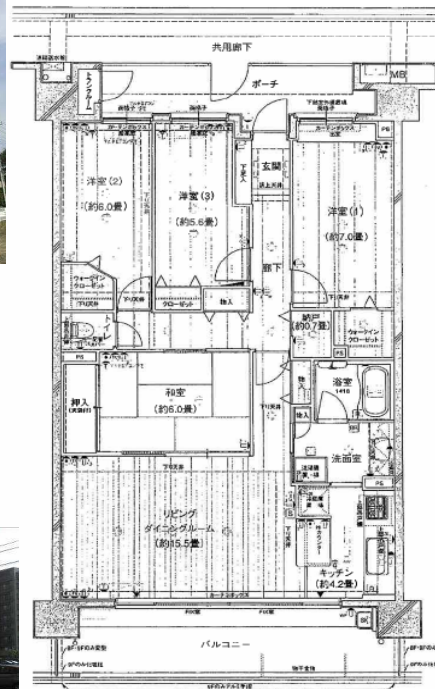
間取り図
